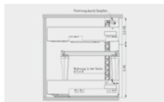
Примеры конструкций с односторонним запираанием
