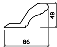
Корона №4 - 2800 x 48 мм Материал: МДФ Основание: 40 мм
