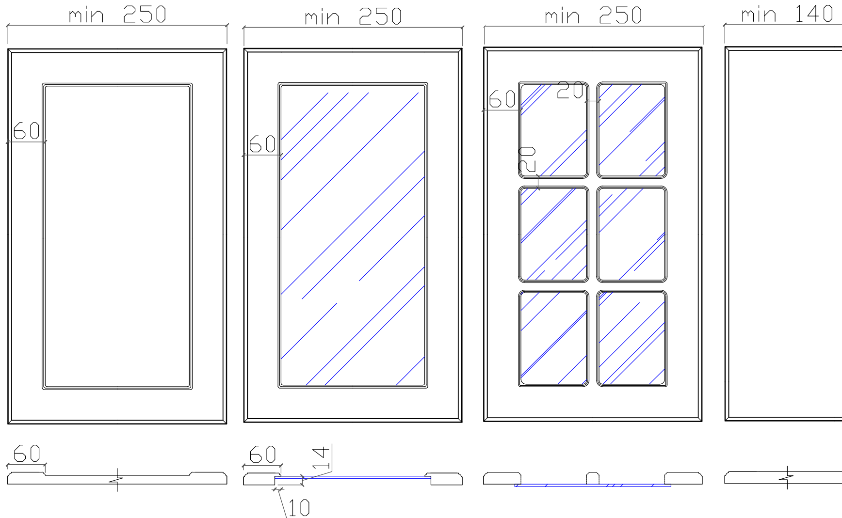
ФАСАД БЕЗ ПРОТОЧЕК
