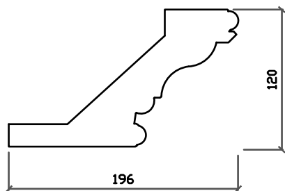
Корона №1 - 3000 x 120 мм Материал: Массив Основание: 110 мм
