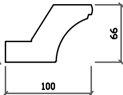
Корона №3 - 3000 x 66 мм Материал: Массив Основание: 60 мм
