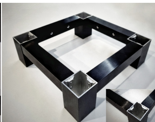
Соединение квадратных труб разных размеров (пример 45x45 с 30x30)
