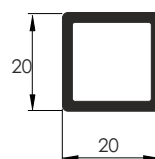
Труба 20x20x2
