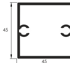
Труба 45x45x1.5 с приливами
