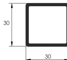
Труба 30x30x2
