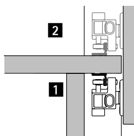
Сторона кріплення, справа
