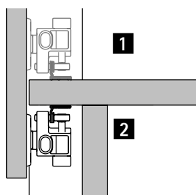
Сторона кріплення, зліва
