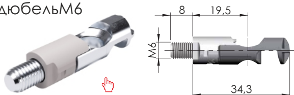
дюбель M6
