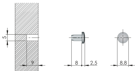
Присадочные размеры
