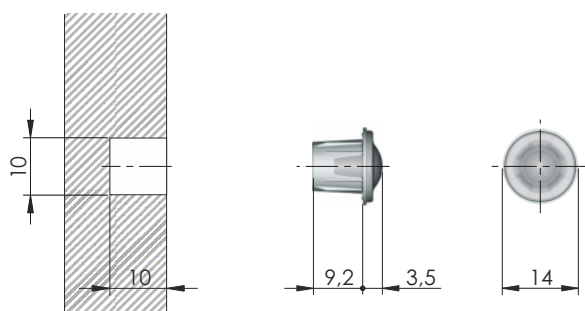
Присадочные размеры
