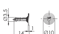
саморез
