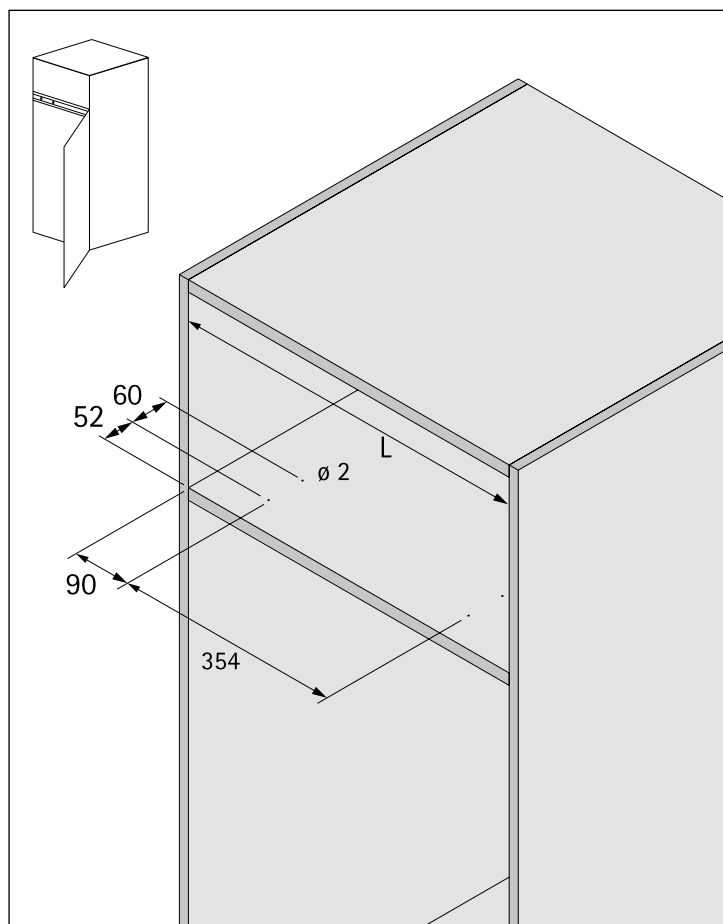
Карта сверления для дверцы холодильника с правой навеской
