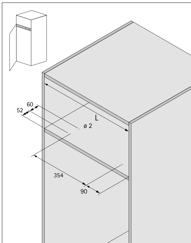
Карта сверления для дверцы холодильника с левой навеской
