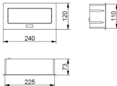
Размерные характеристики
