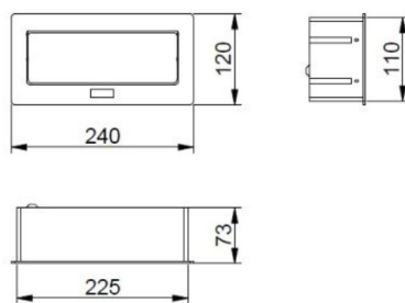
Размерные характеристики
