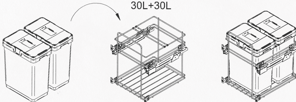
PKBGM453M 30L+10L+9L
